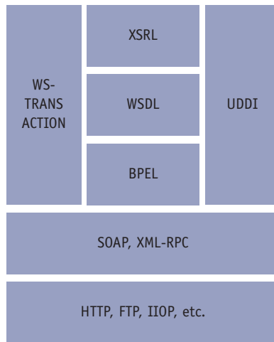
FIGURA 26. Lenguajes y estándares básicos en SOC.
